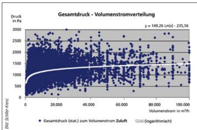
Bild 4 Statistische Verteilung der Gesamtwiderstände (Zuluft).
